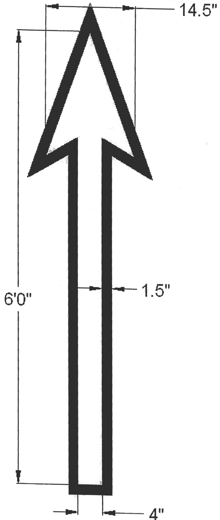
6' Mini Str Arrow W/Cont
